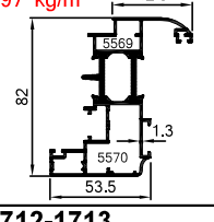
64-1712-1713 1.643 kg/m
