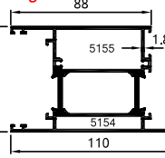
64-4300-4302 2.217 kg/m
