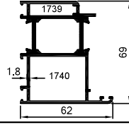
64-1700-1716 1.431 kg/m
