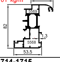
64-1714-1715 1.938 kg/m
