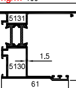
64-5130-5131 1.673 kg/m
