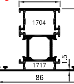
64-5521-5522 2.326 kg/m
