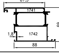
64-1702-1761 1.614 kg/m
