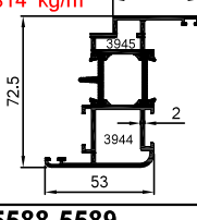
64-5588-5589 1.773 kg/m
